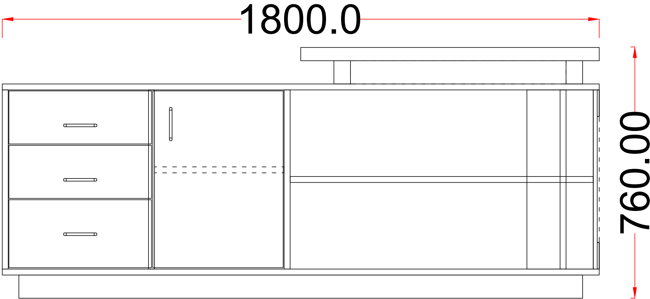
VIEW A-A
